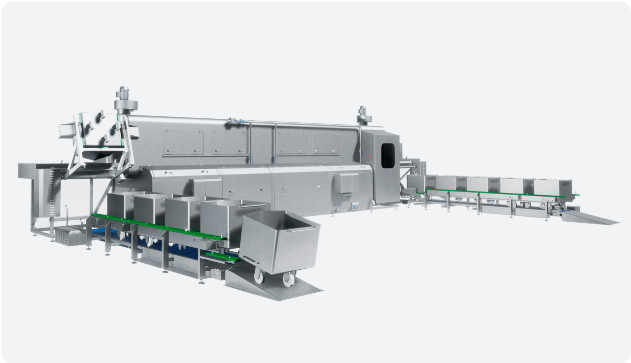
Túnel lavado de bañeras 200L 50-60 u/h 200L Tub washing tunnel 50-60 u/h Tunnel de Lavage de Baignoires 200L 50-60 u/h
